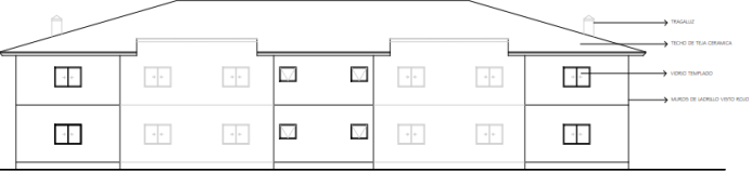
FACHADA POSTERIOR ESC 1/50
