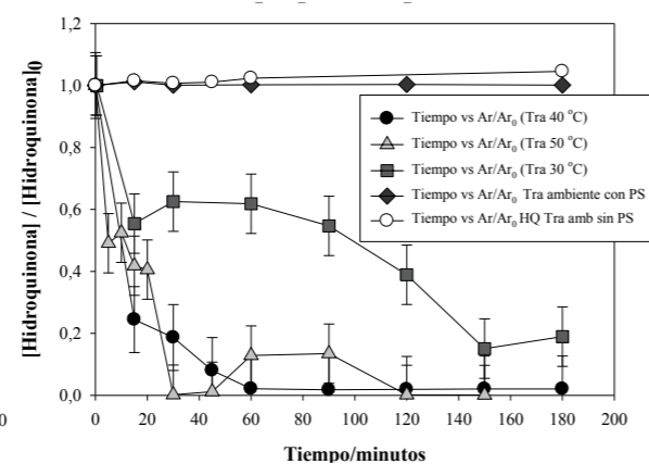
Figura 2. Evolución temporal de concentración para la degradación de hidroquinona a diferentes condiciones experimentales.
