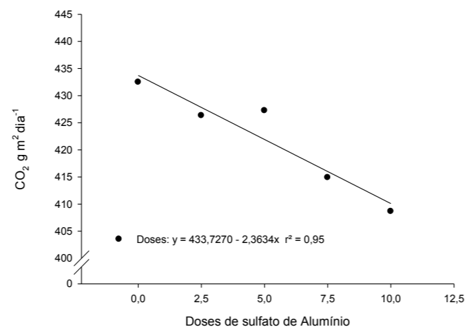
Figura 1. Valores médios da emissão de CO 2 no processo de compostagem de cama de aviário com diferentes doses de aplicação de sulfato de alumínio.
