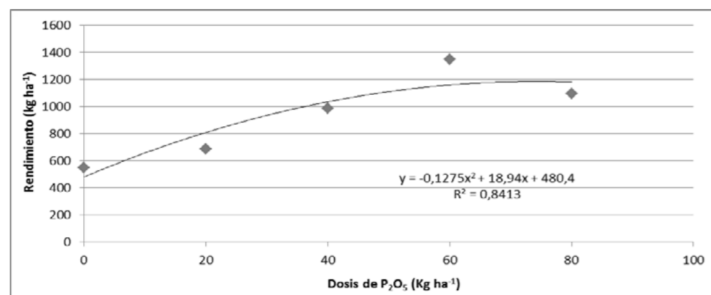
Figura 1. Efecto de la aplicación de fertilizante fosfatado sobre el rendimiento del sésamo variedad escoba.
