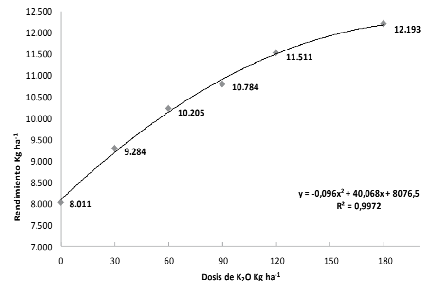
Figura 1. Rendimiento del cultivo de arroz (kg ha -1 ) en función a diferentes dosis de potasio. Caapucú. Paraguari, 2013.
