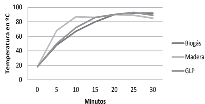
Figura 1. Variación de la temperatura del agua pura
