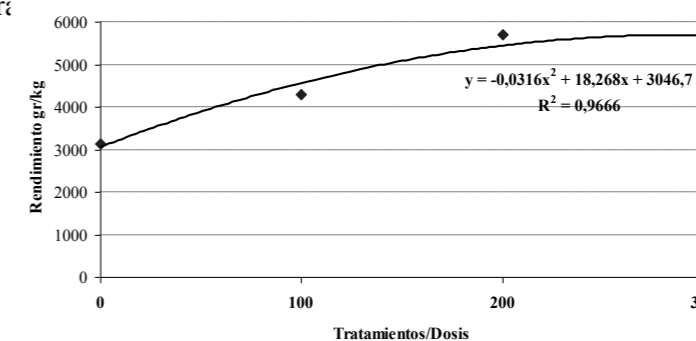
Figura 2. Curva ajustada del rendimiento de forraje verde hidropónico.
