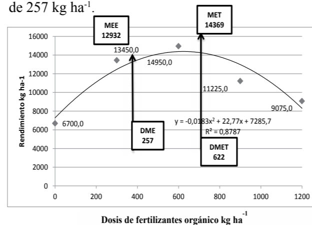
Figura 2. Ecuación del rendimiento del cultivo de jengibre.
