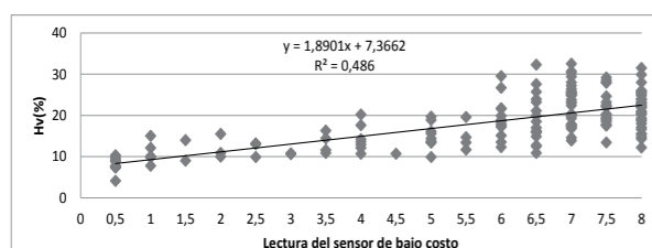
Figura 1. Lecturas de humedad volumétrica (Hv) vs Lecturas del sensor de bajo costo
