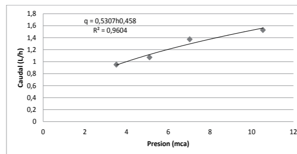
Figura 1. Relación de la Curva Caudal vs Presión del emisor Silver drip .
