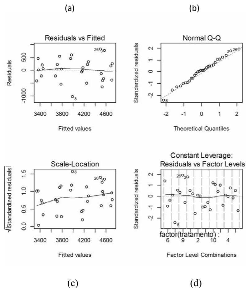
Figura 1. Gráficos de diagnóstico: a) resíduos do modelo ajustado em relação aos valores preditos b) quantis teóricos da distribuição normal padrão em relação aos quantis observados c) resíduos padronizados em relação aos valores ajustados d) avaliação de pontos influentes.
