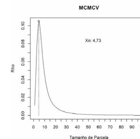
Figura 1. Relação entre curvatura e tamanho de parcela X de um ensaio em branco com mandioca.
