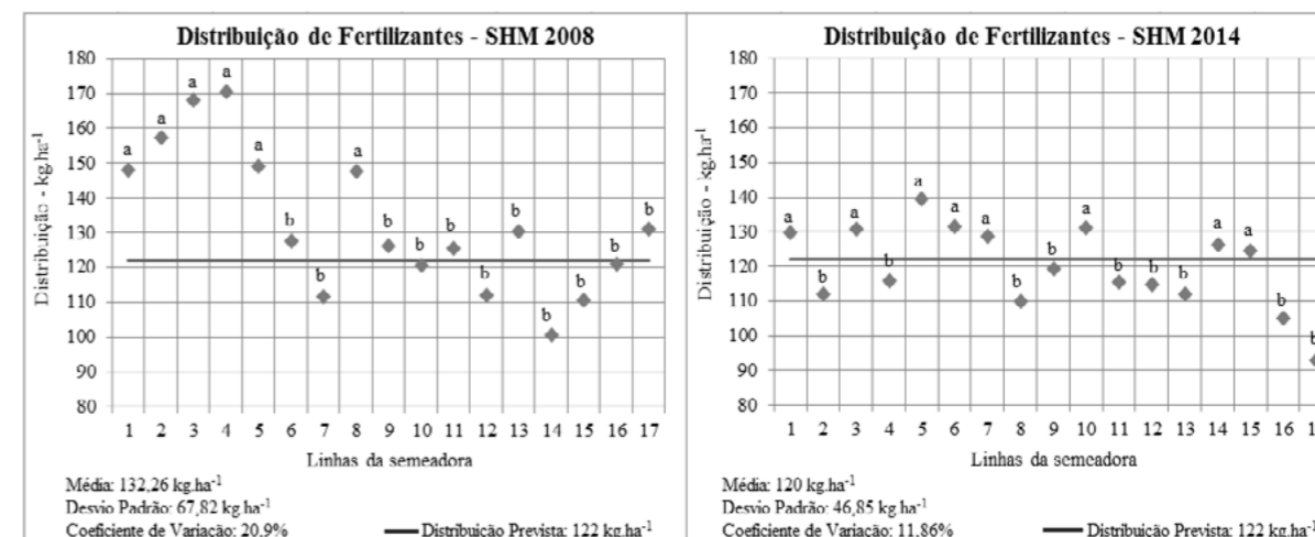
Figura 1. Comparação na distribuição de fertilizantes (NPK) entre duas semeadoras de arrasto com diferentes idades de uso. Dois Vizinhos, Paraná, 2014.
