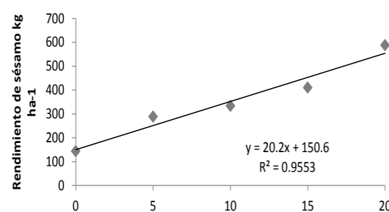
Figura 1. Rendimiento de granos de sésamo en función a diferentes dosis de estiércol bovino. Eusebio Ayala, Cordillera. 2011.
