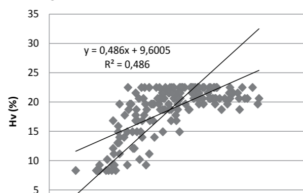
Figura 2. Dispersión de los valores calculados de humedad volumétrica en torno a la recta 1:1 de humedad volumétrica correspondiente a las lecturas de Hidro Farm
