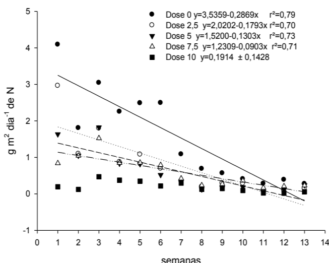
Figura 1. Perda de nitrogênio durante o processo de compostagem de cama de aviário com diferentes doses de aplicação de sulfato de alumínio.
