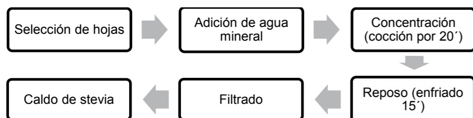
Figura 1. Flujograma de proceso de obtención del caldo de Stevia
