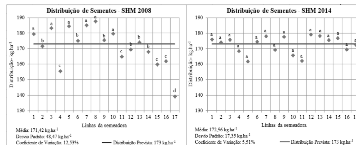
Figura 2. Comparação na distribuição de sementes de trigo entre duas semeadoras de arrasto com diferentes idades de uso. Dois Vizinhos, Paraná, 2014.
