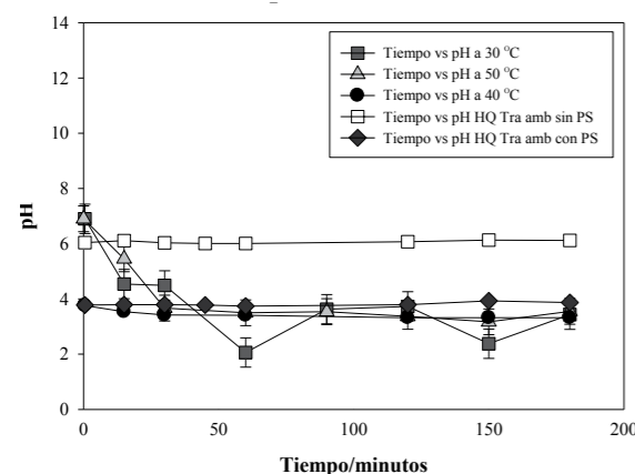
Figura 1. Evolución temporal del pH para la degradación de hidroquinona a diferentes condiciones experimentales.
