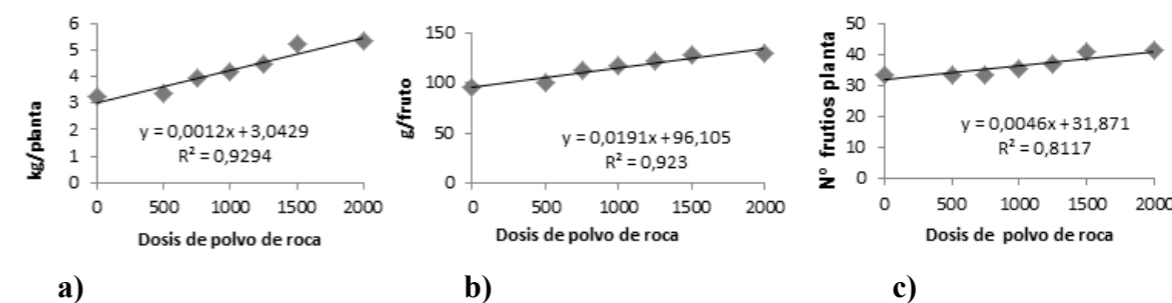
Figura 1. Curva de regresión ajustada para rendimiento de frutos (a), masa de frutos (b) y número de frutos por planta de tomate (c), en función a las dosis de polvo de roca.
