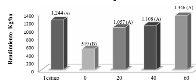
Figura 1. Efecto de diferentes momentos de asociación de kumanda vyvra'í sobre el rendimiento del maíz. Medias con una letra común no son significativamente diferentes ( p \leq 0,05 ). FCA-UNA-Filial Caazapá, 2011.
