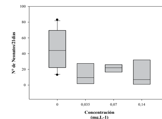
Figura 1. Diagrama de cajas de los números de neonatos de D. magna a diferentes concentraciones de Mancozeb.
