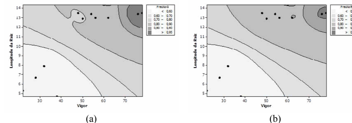
Figura 1. Gráfico de contorno dos modelos de regressão Gama (a) e Beta (b).
